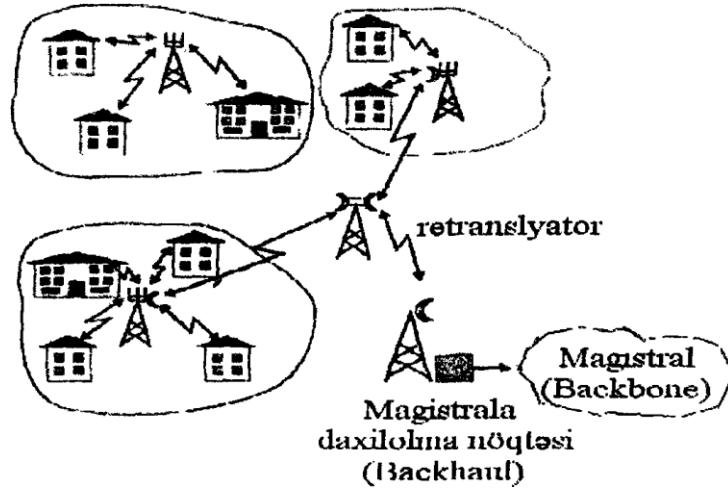
WiMAX şəbəkəsinin arxitekturası
