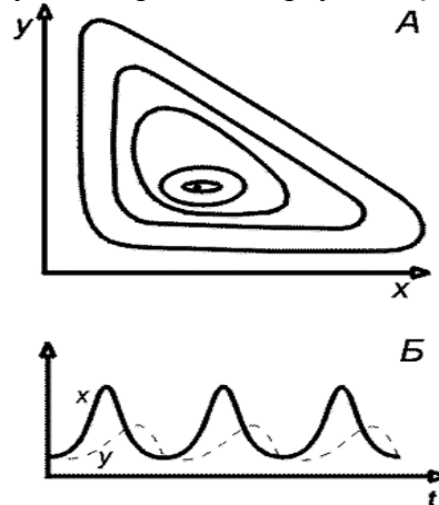
Şəkil 1. Volterin yırtıcı-qurban modeli. A. Baçlanğıc (faza) portreti. B. Qurban və yırtıcı sayının zamandan asılılığını ifadə edir [4].
